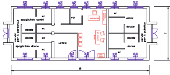
Locale Uffici / Servizi mq 126,00
